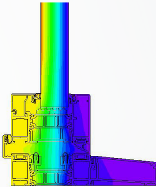
F80 THERMAL PROFILE
